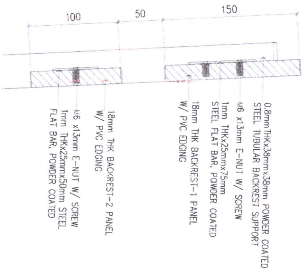
3 DETAIL - 1 1 : 50 M
