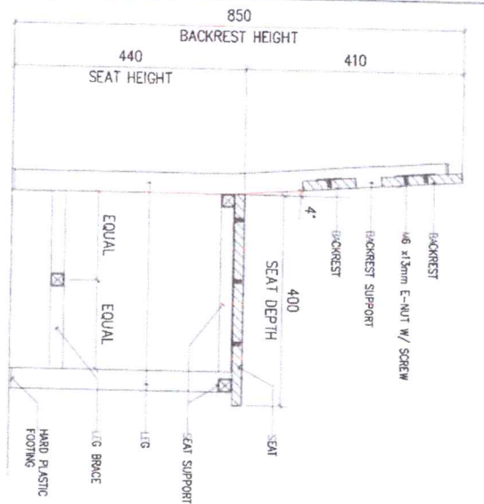
1 CROSS SECTION 1 : 50 M
